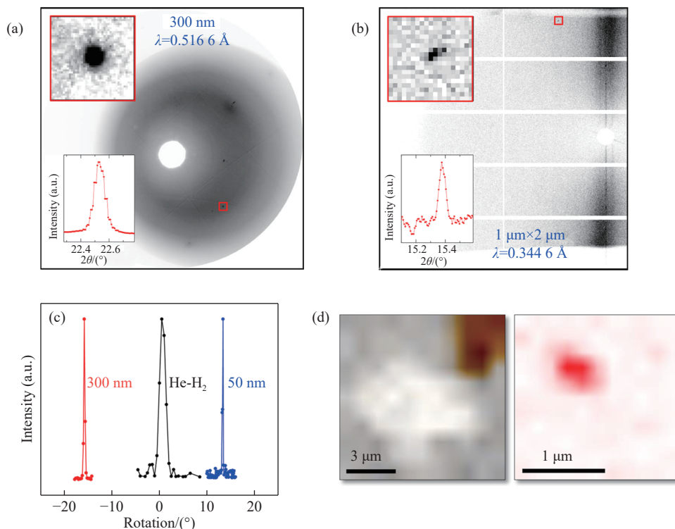
图 4 300 nm 聚焦光束、MCC 采集 X 射线衍射数据结果: (a) MarCCD165 探测器采集数据, (b) Pilatus 1M 探测器采集数据, (c) 不同实验条件的摇摆曲线对比, (d) X 射线衍射对比度成像结果(左图为二维扫描采集的样品 X 射线衍射对比度成像,灰色代表氧化镁衍射峰,橙色代表金的衍射峰,白色区域为氢;右图为氢晶粒的 X 射线衍射对比度成像,红色代表氢的衍射峰强弱)
