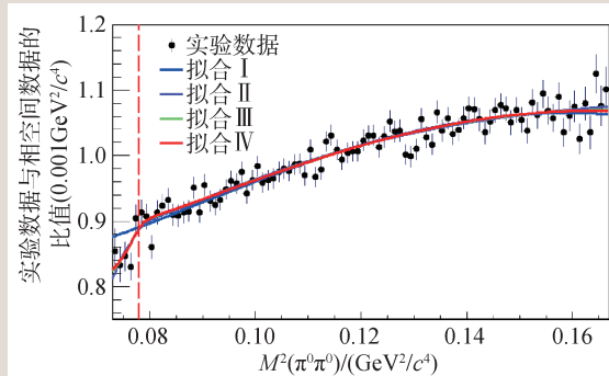
图4 \pi^0 \pi^0 不变质量的分布，其中虚线用于标识 \pi^+ \pi^- 质量阈值之处的拐点效应
