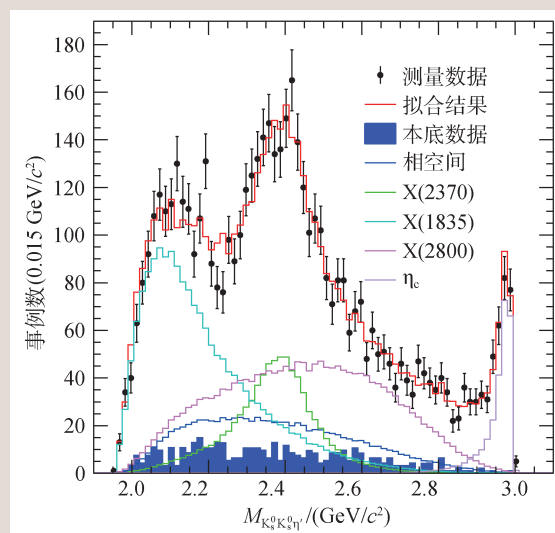
图1 类胶球(glueball-like)粒子X(2370)的发现
