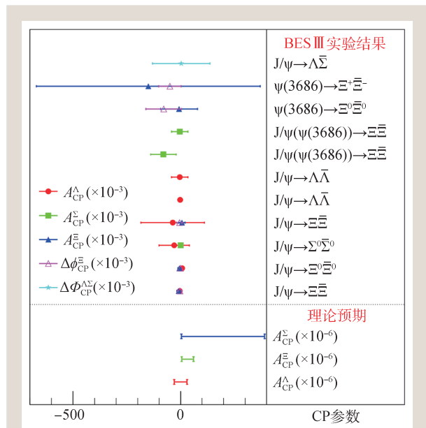
图3 北京谱仪Ⅲ实验上的电荷宇称不对称性检验。其中,左侧图中不同的符号代表不同的CP破坏变量,符号宽窄代表当前测量结果的误差大小。右侧标注的是 BESⅢ实验所采用的不同的衰变过程。图中虚线下方是当前理论预言的CP破坏变量的大小
