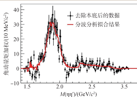
图2 BESⅢ首次发现同位旋标量 1^{-+} 奇特强子态 \eta_1(1855)
