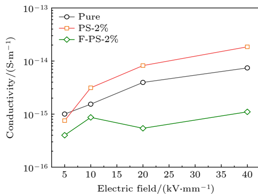
图 5 Pure EP, PS-EP 和 F-PS-EP 在不同场强下的电导率
