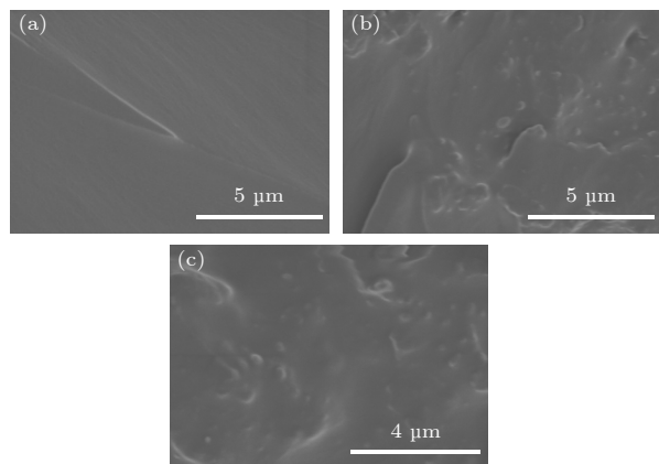
图 3 (a) Pure EP、(b) 填充 PS 和 (c) F-PS 纳米微球后环氧树脂复合材料断面形貌
