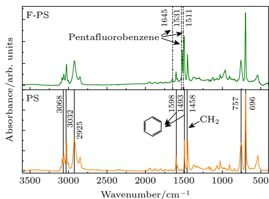
图 2 氟化前后的 PS 纳米微球的 FT-IR 图谱.
