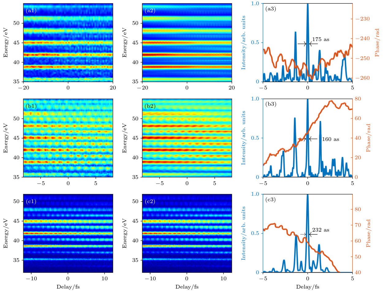
图 5 FROG-CRAB 反演实验 RABBITT 能谱图重建阿秒脉冲串结果 (a1), (b1), (c1) 实验测到的 3 组 RABBITT 能谱图; (a2), (b2), (c2) 根据反演脉冲重建的能谱图; (a3), (b3), (c3) 反演得到的时域阿秒脉冲串和相位
