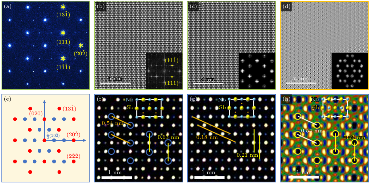
图 5 (a) Nb 0.84 CoSb [110] 取向的选区电子衍射花样; (b) Nb 0.84 CoSb [110] 取向的滤波像; (c), (d) 分别仅包含主衍射点信息和超结构衍射信息的滤波像; (e) Nb 0.84 CoSb 超结构衍射点示意图; (f)–(h) 图 (b)–(d) 的放大像
