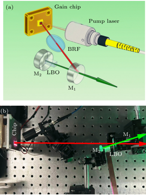
图 2 (a) 倍频绿光 VECSEL 的 V 型谐振腔结构图; (b) 实验装置实物图
