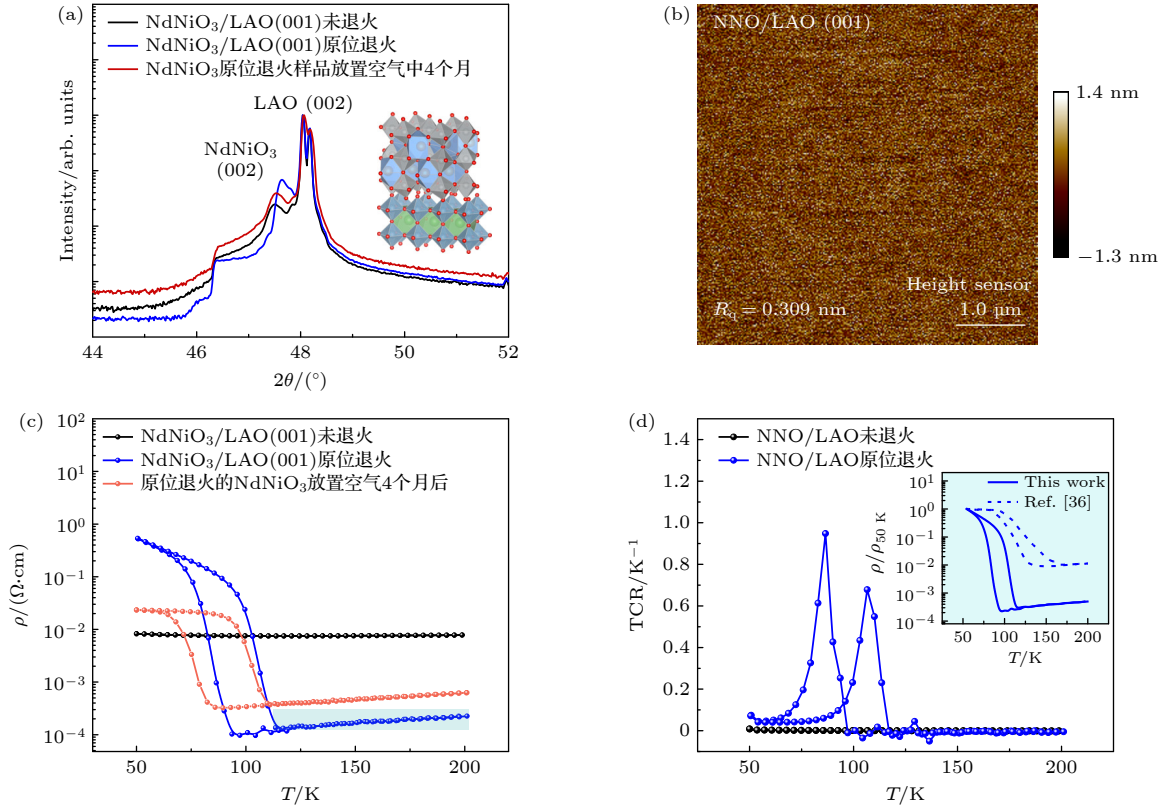
图 2 揭示高氧压原位退火在沉积 \text{ReNiO}_3 薄膜中的关键作用 (a) 未经原位退火、经原位退火及放置空气中 4 个月后 \text{NdNiO}_3 的 X 射线衍射图谱 (XRD); (b) 经原位退火 \text{NdNiO}_3 薄膜的原子力显微镜 (AFM) 图; (c) 原位退火、放置于空气中 4 个月及未经原位退火 \text{NdNiO}_3 的阻温特性曲线 ( \rho - T 曲线); (d) 原位退火及未经原位退火 \text{NdNiO}_3 的电阻温度系数与温度的变化关系图 (TCR - T 曲线), 插图为本工作制备的 \text{NdNiO}_3 薄膜的归一化特性曲线与文献 [36] 的对比图
