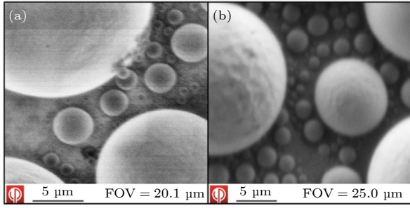
图 14 拍摄的碳衬底上锡球的图像比较 (a) 束流能量 5 keV, 束流电流 7 pA 的 Cs + -FIB; (b) 束流能量 5 keV, 束流电流 20 pA 的商业化产品 Ga-LMIS FIB [50]
