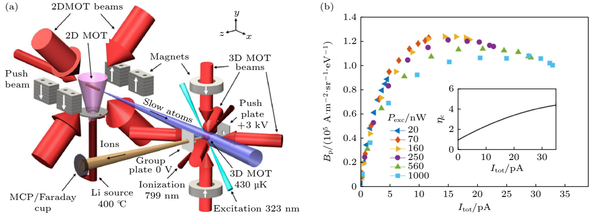
图 12 (a) Li-MOTIS 装置示意图; (b) 不同紫外激发功率 ( P_{\text{exc}} ) 下离子源亮度 ( B_p ) 与束流流强 ( I_{\text{tot}} ) 的关系 [47]
