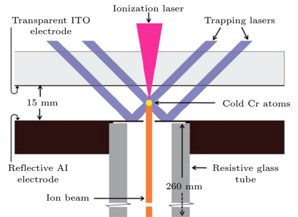
图 10 Cr-MOTIS 装置示意图 [43]
