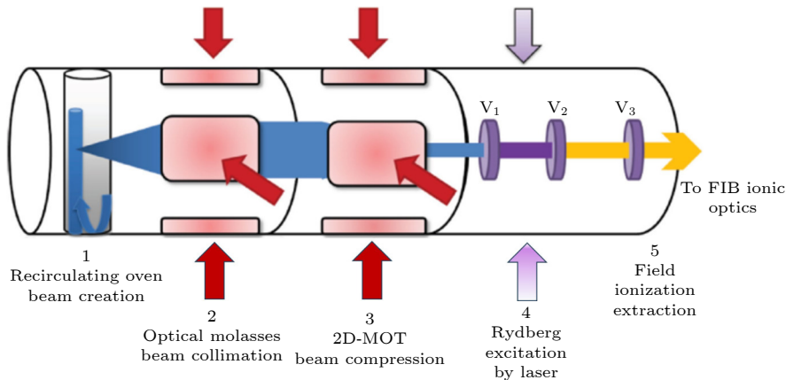
图 13 场电离里德伯态原子方案的 CABIS 装置结构示意图 [23] , 利用 2D-MOT 技术对高通量原子束进行横向冷却和压缩, 离子或电子 (取决于电极的极性) 由场电离冷里德伯态原子产生, 之后束流在 FIB 系统中被加速和聚焦
