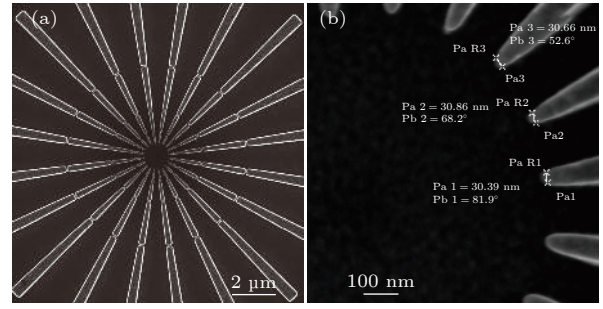
图 7 (a) 分辨率测试卡中央的西门子星结构的 SEM 图像; (b) 西门子星最内环局部结构的 SEM 图像
