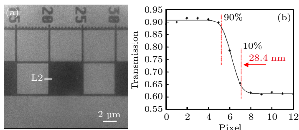
图 9 刀口测试结果 (a) 刀口的 TXM 图像; (b) L2 处的刀口响应曲线
