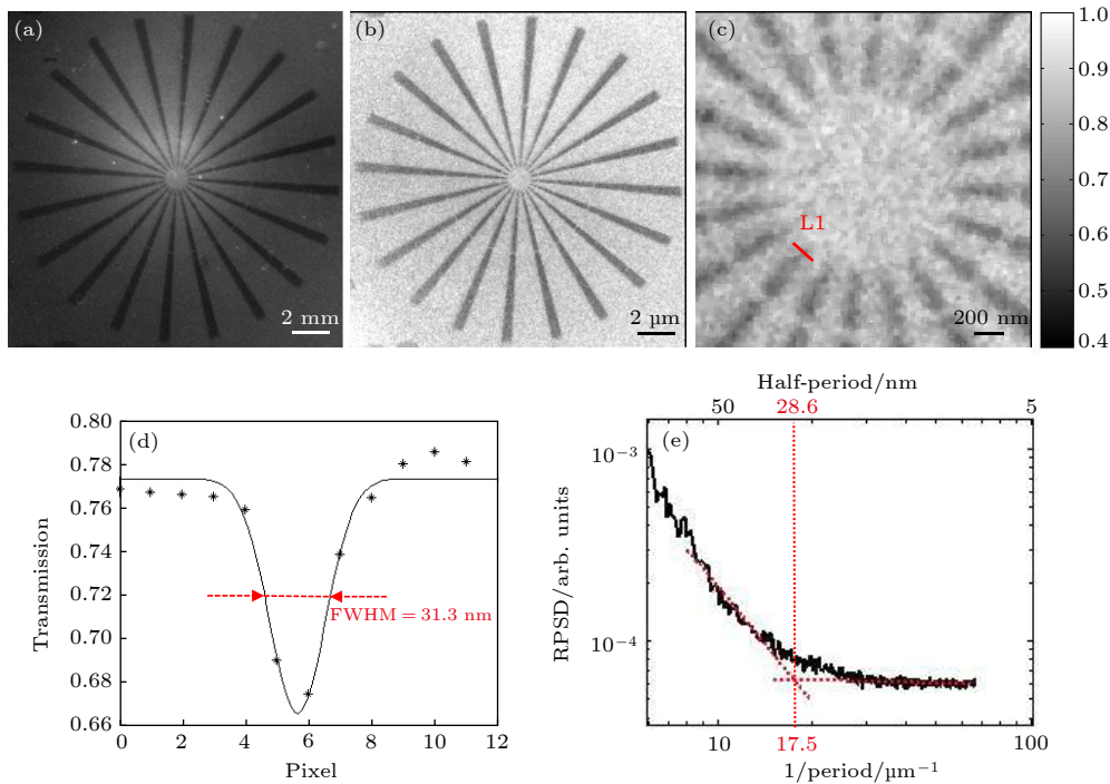
图 8 分辨率测试卡 TXM 测试结果 (a) 西门子星结构的 TXM 图像; (b) 扣除背底后的西门子星结构的透过率图像; (c) 西门子星结构的内环结构局部放大图; (d) 30\ \text{nm} 线宽的栅条结构的透过率分布曲线; (e) 径向功率谱强度曲线
