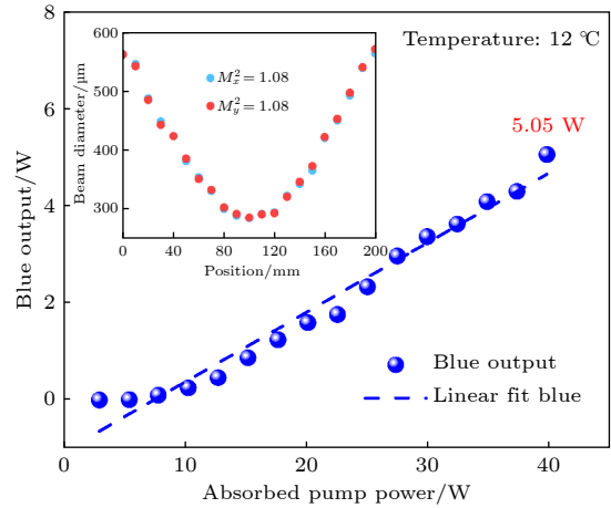
图 5 VECSEL 的 M^2 因子测量图及功率曲线
