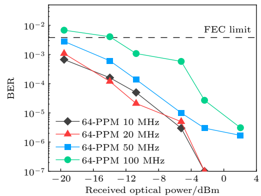
图 11 64 PPM 在不同带宽频率下的误码率与接收光功率的关系
