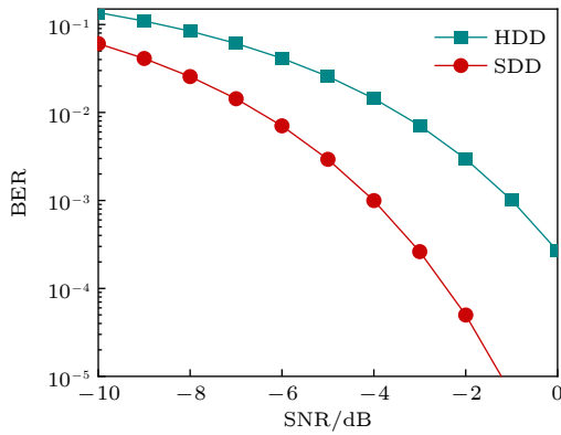
图 9 硬判决与软判决误码率仿真
