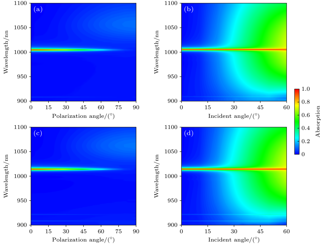
图 9 w = 155 nm 时, (a) 光源偏振角 \alpha 和 (b) 光源入射角 \theta 对 BIC 的影响; 分别是 w = 140 nm 时, (c) 光源偏振角 \alpha 和 (d) 光源入射角 \theta 对 BIC 的影响
