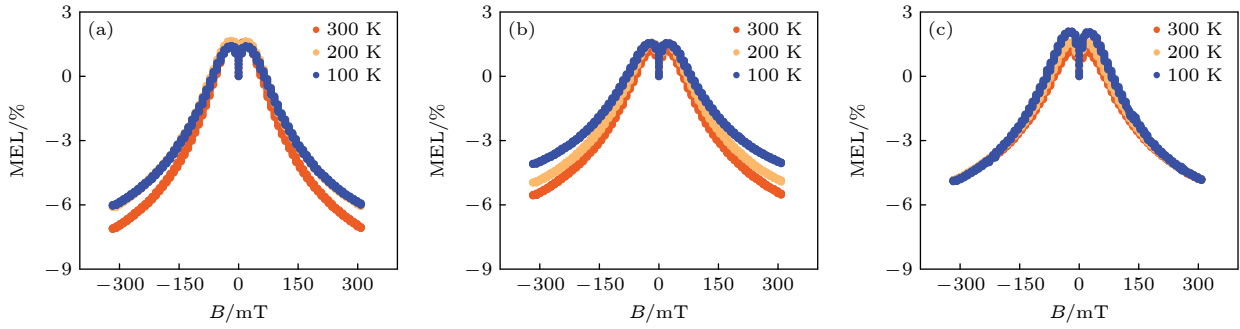
图 6 (a)–(c) 电流 500 \mu\text{A} 时器件 1–3 中温度依赖的 MEL 曲线
