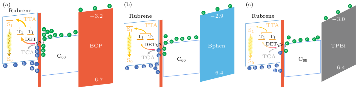
图 3 (a)–(c) 器件 1–3 的微观机理示意图
