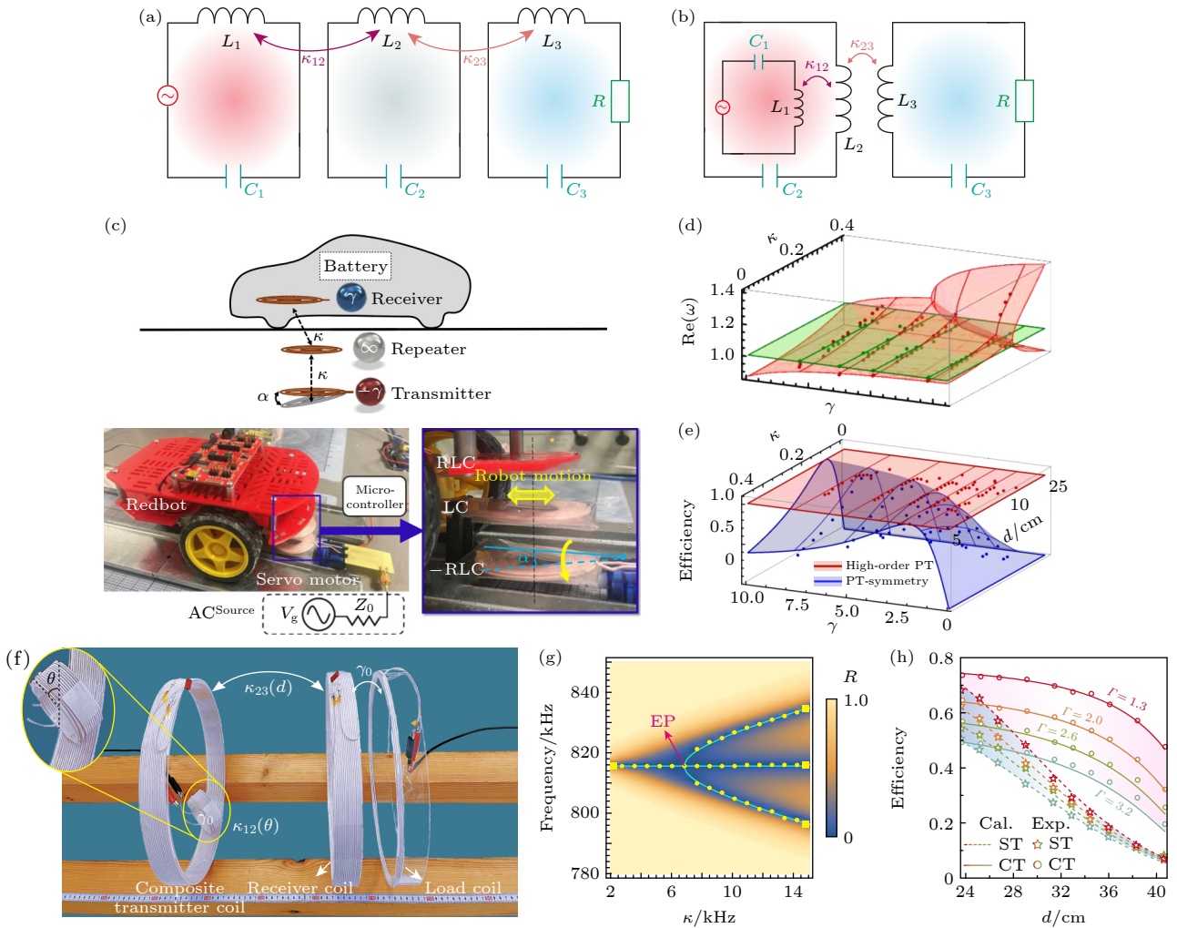
图 5 三阶 PT 对称 WPT 系统的实现 (a) 分离型三阶系统电路图; (b) 合成型三阶系统电路; (c) 小车三阶 WPT 演示图 [23]; (d) 三阶系统实部随耦合和损耗的演化轨迹 [23]; (e) 理想情况下三阶和二阶系统效率对比图 [23]; (f) (b) 图对应实验图 [38]; (g) 三阶系统反射率随频率和耦合强度的变化关系 [38]; (h) 不同本征损耗下效率与传输距离变化图 [38]
