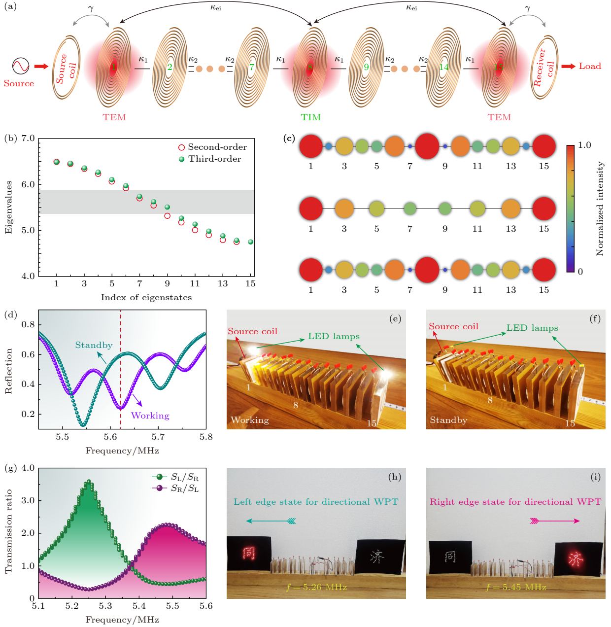
图 10 (a) PT 对称的多线圈复合二聚链 WPT 系统示意图 [59] ; (b) 等效三阶 PT 对称 (绿色) 和等效二阶 PT 对称 (橙色) 拓扑二聚体链的特征值谱 [59] ; (c) 等效三阶 PT 对称的复合拓扑二聚体链中的三种拓扑模式的归一化强度分布 [59] ; (d) 拓扑二聚体链在工作 (红色) 和待机 (蓝色) 状态下的反射谱 [59] ; (e) 图 (d) 在工作状态下实验演示 [59] ; (f) 图 (d) 在待机状态下实验演示 [59] ; (g) 一维 Harper 链左右两端的传输比 [60] ; LED 灯组成汉字的“同”和“济”的定向 WPT 的演示实验 (h) 左向演示 [60] ; (i) 右向演示 [60]
