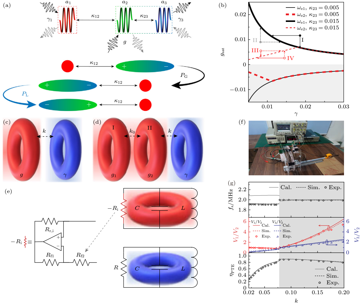
图 7 (a) 基于偶极-单极类比的广义奇偶性的局部和全局奇偶性分解 [41] ; (b) 高维参数空间 (g, \gamma, \kappa_{12}, \kappa_{23}) 中 WPT 系统的能带理论解释 [41] ; (c) 标准 PT 对称电子二聚体的示意图 [42] ; (d) 由两个增益 (红色) 单元和一个损耗 (蓝色) 单元组成的三阶赭厄密系统 [42] ; (e) 增益单元和损耗单元对应的等效电路 [42] ; (f) 图 (d) 模型的实验装置示意图 [42] ; (g) 稳态频率 f_s (上图), 电压比 V_1/V_2 (左侧红色 y 轴) 和 V_3/V_2 (右侧蓝色 y 轴) (中间图), 以及传输效率 \eta_{\text{PTE}} (下图), 作为耦合系数 \kappa 的函数. 理论, 模拟和实验结果分别用实线、虚线和空心圆表示. 阴影区域表示 \kappa \geq \gamma = 0.078 [42]
