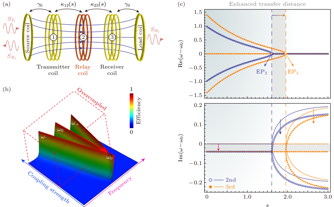
图 4 三阶 PT 对称 WPT 系统 [38]: (a) 三阶 PT 对称模型图; (b) 三阶 PT 对称系统效率随频率和耦合强度变化关系; (c) 二阶和三阶 PT 对称系统传输实部虚部相图对比
