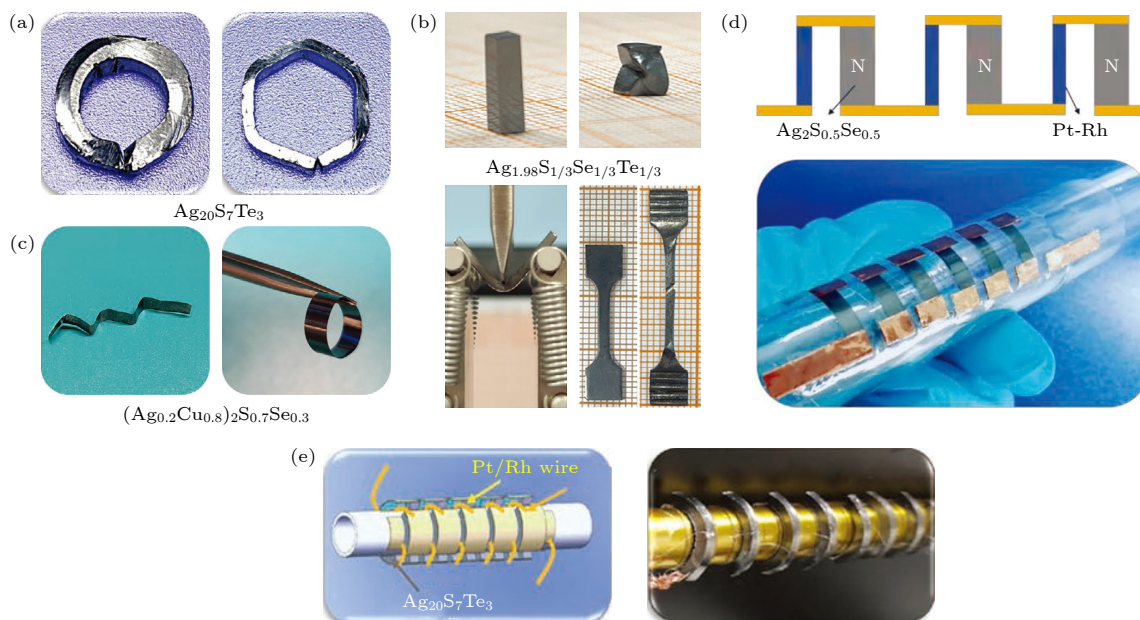
图1 \text{Ag}_2\text{S} 基塑性热电材料 (a) \text{Ag}_{20}\text{S}_7\text{Te}_3 [12]; (b) \text{Ag}_{1.98}\text{S}_{1/3}\text{Se}_{1/3}\text{Te}_{1/3} [15]; (c) (\text{Ag}_{0.2}\text{Cu}_{0.8})_2\text{S}_{0.7}\text{Se}_{0.3} [16]; 基于 \text{Ag}_2\text{S}_{0.5}\text{Se}_{0.5} (d) 和 \text{Ag}_{20}\text{S}_7\text{Te}_3 (e) 的塑性热电器件[10,12]. 引用的图片已获相关授权
