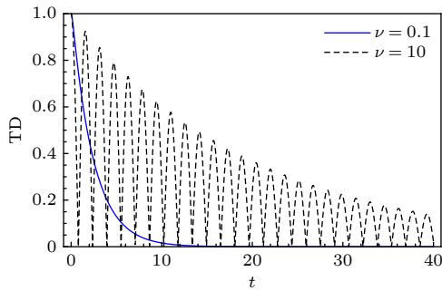
图 1 迹距离 TD 随时间的演化
