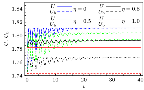
图 5 初态为可分离态时, 熵不确定度 U 及其下限 U_b 随时间的演化. 通道参数 \nu = 10 , 呈现非马尔科夫性
