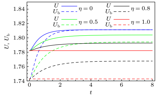
图 4 初态为可分离态时熵不确定度 U 及其下限 U_b 随时间的演化. 通道参数 \nu = 0.1 , 呈现马尔科夫性
