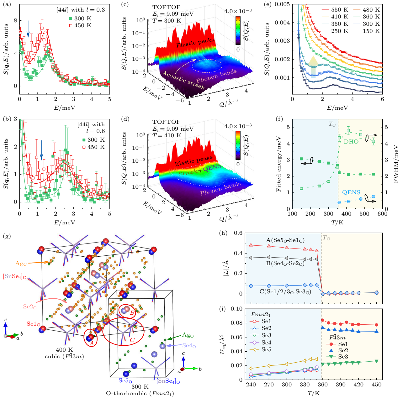
图 9 \text{Ag}_3\text{SnSe}_6 超离子相变过程中的晶格动力学与亚晶格耦合行为 [31] (a), (b) 在日本 J-PARC 中子源的 AMATERAS 谱仪测得的 300 K 和 450 K 温度下, [4 4 0.3] 和 [4 4 0.6] TA 声子模的实验数据; (c), (d) 在德国 FRM II 中子源的 TOFTOF 直接几何谱仪测得的 \text{Ag}_3\text{SnSe}_6 多晶样品在 300 K 和 410 K 的动力学结构因子 S(Q, E) ; (e) 在 [2.0, 2.4] \text{\AA}^{-1} 的动量 Q 范围内对 S(Q, E) 进行积分获得的动力学结构因子曲线; (f) 通过对图 (e) 中的曲线进行阻尼谐振子模型和洛伦兹模型拟合获得的声子能量、半高宽和 QENS 信号展宽; (g) 法国 ILL 中子源 D9 单晶中子衍射谱仪上获得的 300 K 和 400 K 下的正交结构 (O) 和立方结构 (C) 的对比; (h), (i) 通过精修原位 XRD 衍射谱获得的 A, B, C 位置的 Se 原子在超离子相变过程中的原子坐标位移 |L| 和各向同性原子位移参数 U_{eq} 的变化, A 对应低温相的 Se5 和高温相的 Se1, B 对应低温相的 Se4 和高温相的 Se2
