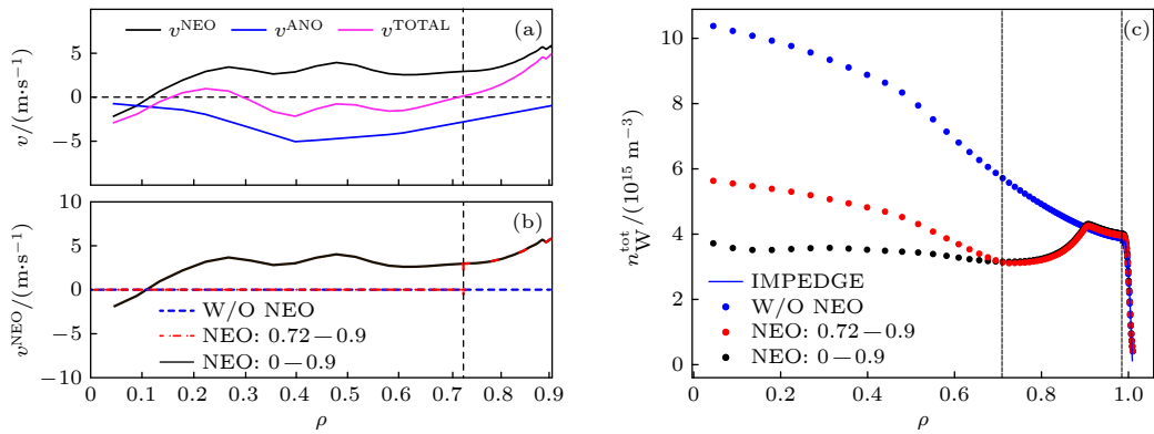
图 4 区域 \rho = 0-0.9 (a) v^{\text{NEO}} , v^{\text{ANO}} 和 v^{\text{TOTAL}} 径向分布; (b) 3 种情况下 v^{\text{NEO}} 分布设置; (c) 区域 \rho = 0-1.01 三种情况下模拟得到的钨杂质密度 n_{\text{W}}^{\text{tot}} 径向分布, 其中杂质边缘分布均与 IMPEDGE 一致, 虚线分别表示 \rho = 0.72 和 \rho = 0.98 所在位置
