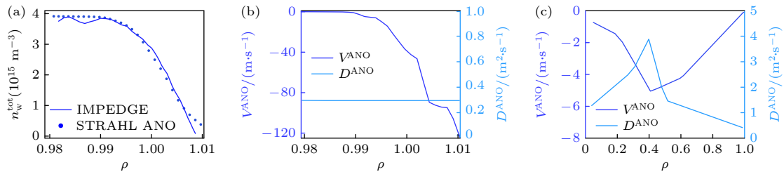
图 3 (a) \rho = 0.98 —1.01 区域的杂质分布, 其中蓝线为 IMPEDGE 模拟分布, 蓝点为 STRAHL 模拟分布; (b) \rho = 0.98 —1.01 区域湍流扩散系数 D^{\text{ANO}} 与对流速度 v^{\text{ANO}} 分布; (c) \rho = 0 —0.98 区域湍流扩散系数 D^{\text{ANO}} 与对流速度 v^{\text{ANO}} 分布
