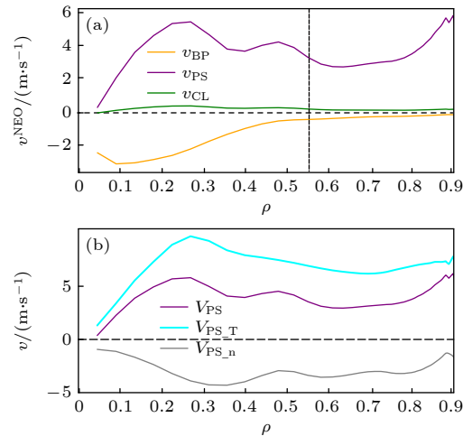
图 5 区域 \rho = 0 - 0.9 (a) 新经典对流速度的 3 个分量; (b) 新经典对流 PS 分量 v_{\text{PS}}^{\text{NEO}} 及离子温度梯度项 v_{\text{PS}_T}^{\text{NEO}} 和密度梯度项 v_{\text{PS}_n}^{\text{NEO}} , 虚线位置为 \rho = 0.55
