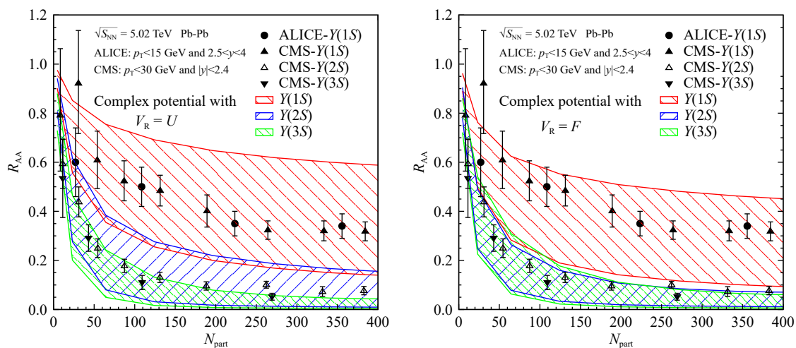
图 4 在 5.02 TeV Pb-Pb 碰撞中, 底夸克偶素 \Upsilon(1S, 2S, 3S) 的核修正因子随着参与碰撞核子数 N_p 的分布 (在线彩图)
