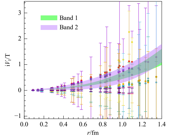
图 1 虚部相互作用势的拟合 (在线彩图)
