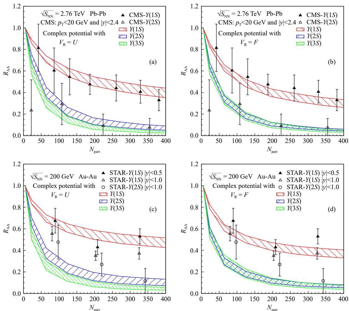
图 3 上面两个图: 在 2.76 TeV Pb-Pb 碰撞中, 底夸克偶素 \Upsilon(1S, 2S, 3S) 的核修正因子随着参与碰撞核子数 N_p 的分布; 下面两个图: 在 200 GeV Au-Au 碰撞中的底夸克偶素核修正因子 (在线彩图)
