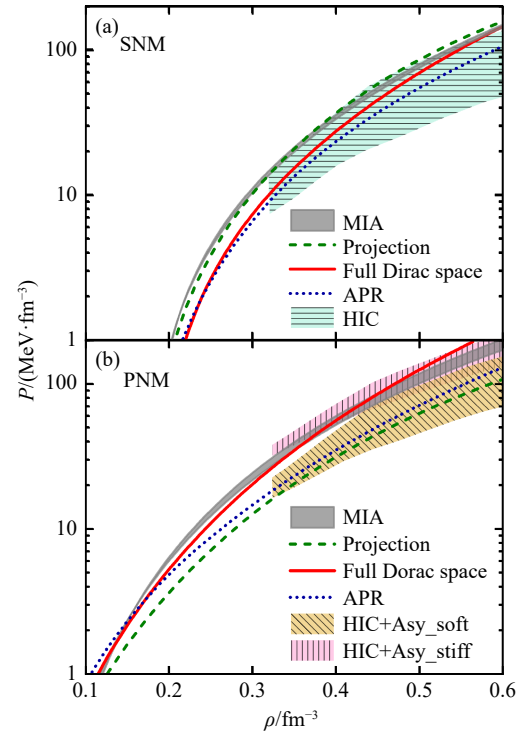
图 7 完备 Dirac 空间的 RBHF 理论计算得到的对称核物质 (a) 与纯中子物质 (b) 的压强 P 随密度 \rho 的变化 (红色实线), 以及与投影方法 (绿色点虚线)、动量无关近似方法 (灰色阴影)、非相对论变分计算 (APR) 和基于重离子碰撞流数据所提取的约束 (HIC) [47] 的对比 (在线彩图)
