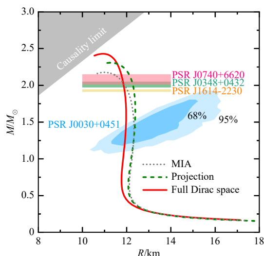
图 10 完备 Dirac 空间的 RBHF 理论计算得到的中子星质量-半径关系(红色实线)、与投影方法(绿色虚线)、动量无关近似方法(灰色点线)的对比(在线彩图)
