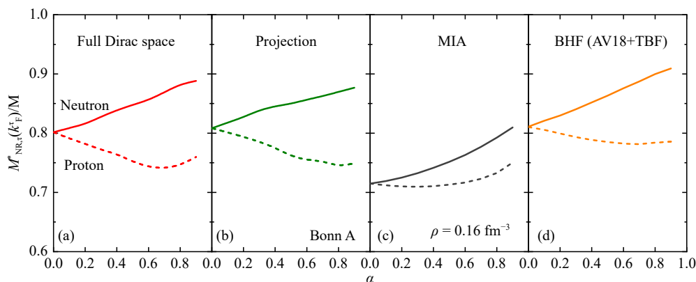
图 5 完备 Dirac 空间的 RBHF 理论计算得到的非相对论有效质量随同位旋不对称度的变化 (a), 以及与投影方法 (b) 和动量无关近似方法 (c) 所得结果的比较。图中还给出了基于 AV18 和微观三体势 (TBF), 非相对论 BHF 的计算结果 (d) [43]
