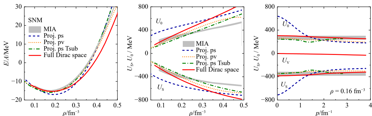
图 3 完备 Dirac 空间的 RBHF 理论得到的核物质结合能和单粒子势 (Full Dirac space), 以及与动量无关近似 (MIA) 和投影方法 (Proj.) 的对比 [37]
