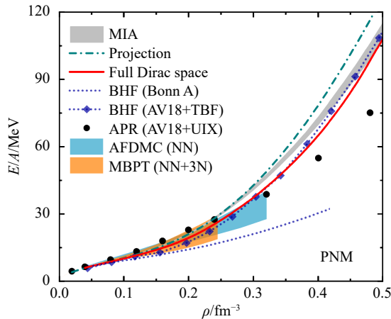
图 6 完备 Dirac 空间的 RBHF 理论计算得到的纯中子物质的每核子结合能随密度的变化 (红色实线), 以及与动量无关近似 (灰色阴影) 和投影方法 (绿色虚线) 的比较 [41] (在线彩图)
