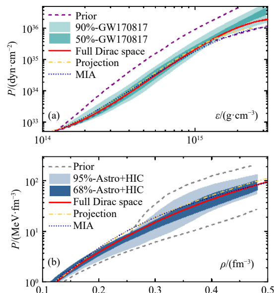
图 9 完备 Dirac 空间的 RBHF 理论计算得到的中子星物质的压强 P 随 (a) 能量密度 \varepsilon 和 (b) 密度 \rho 的变化 (红色实线), 与投影方法 (橙色点虚线)、动量无关近似方法 (蓝色点线)、文献 [55] 基于引力波数据所得约束 (绿色阴影)、和文献 [56] 结合天文观测数据和重离子碰撞数据所得约束 (蓝色阴影) 的对比 [41] (在线彩图)
