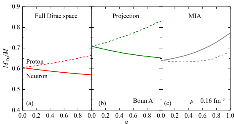
图 4 完备 Dirac 空间的 RBHF 理论计算得到的 Dirac 质量随同位旋不对称度的变化 (a), 以及与投影方法 (b) 和动量无关近似方法 (c) 所得结果的比较 [38]
