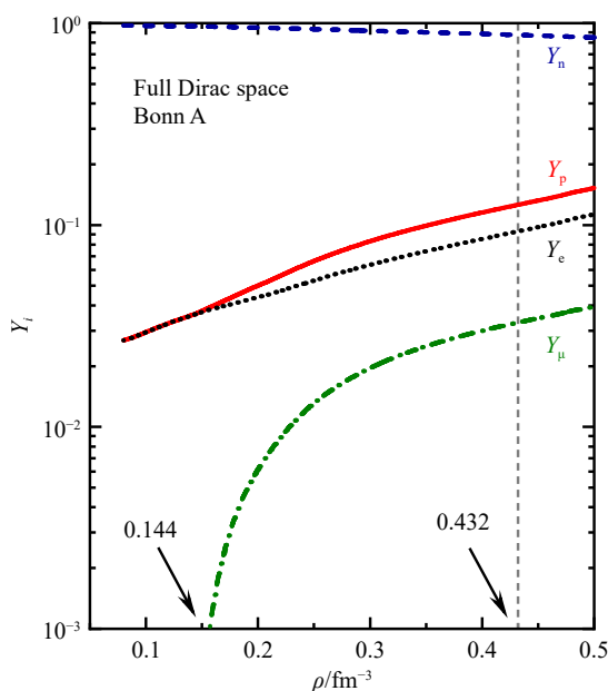
图 8 完备 Dirac 空间的 RBHF 理论计算得到的中子星物质的粒子分数 Y_i ( i = n, p, e, \mu ) 随重子数密度的变化 [39]
