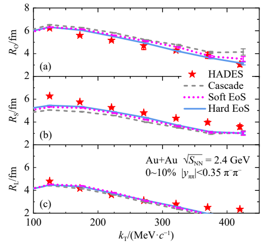
图 3 \sqrt{s_{NN}}=2.4 GeV 下 Au+Au 中心 (0~10%) 碰撞中横动量 k_T 依赖的 HBT 半径 R_O , R_S 和 R_L 。实验数据来自于 HADES 合作组 [28]
