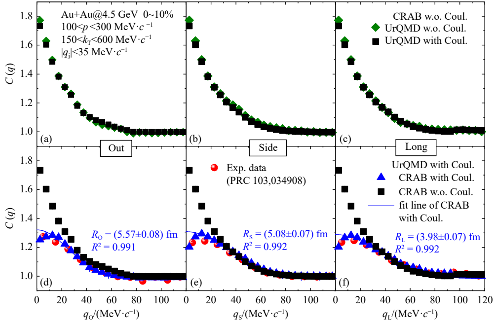
图 2 碰撞能量为 \sqrt{s_{NN}}=4.5 GeV 的 Au+Au 中心 (0~10%) 碰撞中, \pi^+\pi^- 介子对的 HBT 关联函数 (实验数据来自于 STAR 合作组 [29])
