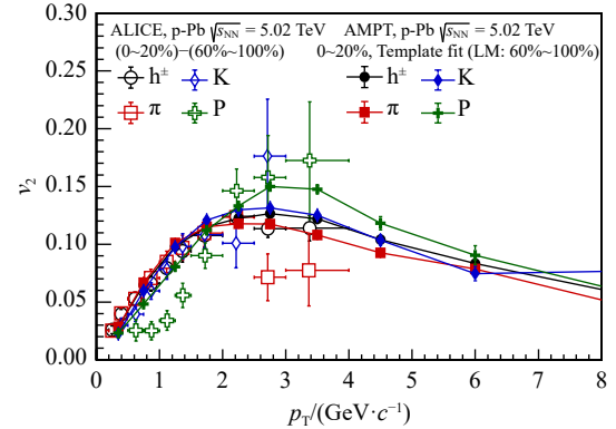
图 2 AMPT 模型在 \sqrt{s_{\text{NN}}} = 5.02 TeV 高多重数 (中心度 0~20%) 的质子-铅核碰撞中对带电强子 h^\pm 、 K^\pm 介子、 \pi^\pm 介子及质子 P(\bar{P}) 的 v_2 的计算结果与 ALICE 的实验观测结果的比较
