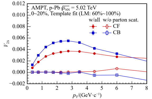
图 5 打开和关闭部分子散射过程的 AMPT 模型在 \sqrt{s_{NN}}=5.02 TeV 质子-铅核碰撞中对带电强子 V_{2d} 随 p_T 分布的计算结果
