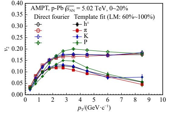
图 1 AMPT 模型在 \sqrt{s_{\text{NN}}} = 5.02 TeV 高多重数 (中心度 0~20%) 的质子-铅核碰撞中对带电强子 h^\pm 、 K^\pm 介子、 \pi^\pm 介子及质子 P(\bar{P}) 的 v_2 随横动量 p_T 分布的计算结果 空心点和实心点分别对应非流效应被减除前与减除后的结果。
