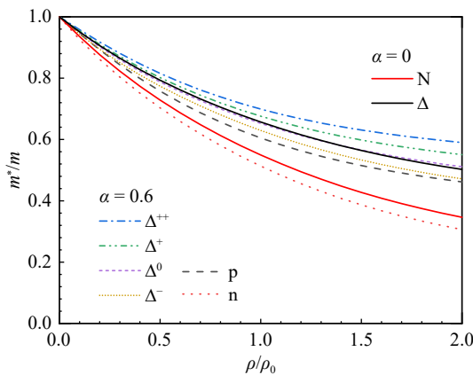
图 1 \alpha=0.6 与 0 时, 核子和 \Delta 粒子有效质量随约化重子密度的变化关系 (在线彩图)
