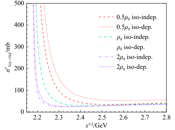
图 2 同位旋不对称度 \alpha=0.6 时, 不同重子密度下同位旋无关和同位旋依赖的 N\Delta \rightarrow N\Delta 的散射截面随质心系能量的变化关系 (在线彩图)
