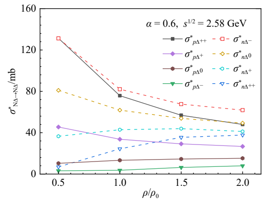
图 3 同位旋不对称度 \alpha=0.6 , 质心系能量为 2.58 GeV 时, N\Delta \rightarrow N\Delta 各分反应道弹性散射截面随重子数密度的变化情况 (在线彩图)
