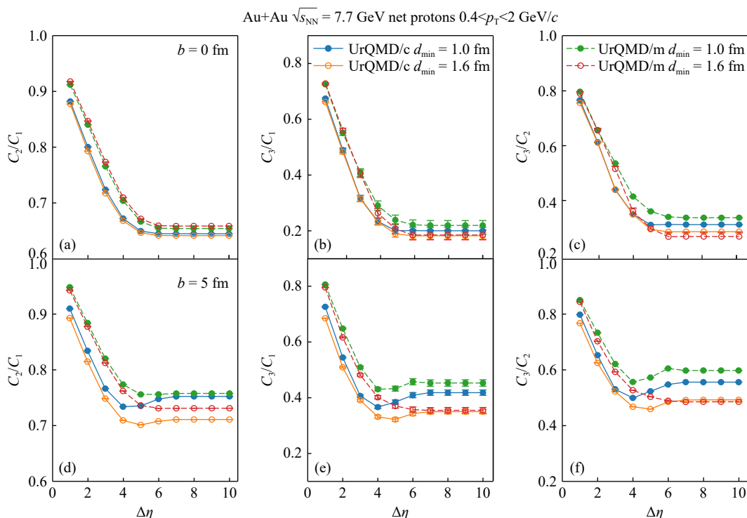
图 5 碰撞参数 b = 0, 5 fm 时, 不同的 d_{\min} 和有无平均场的模式下净质子数的 C_2/C_1 , C_3/C_1 和 C_3/C_2 随赭快度窗口 \Delta\eta 的变化 (在线彩图)
