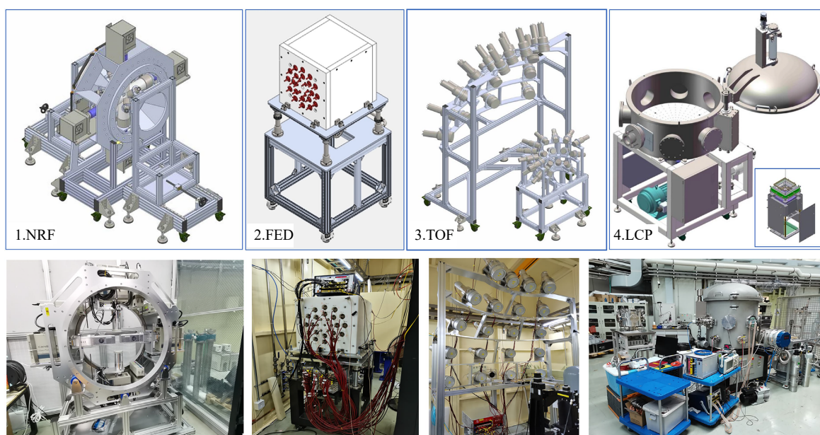
图 3 核共振荧光谱仪 NRF, 平坦效率谱仪 FED, 飞行时间谱仪 TOF 和轻带电粒子谱仪 LCP 的工程制图 (上图) 和对应的现场照片 (下图)
