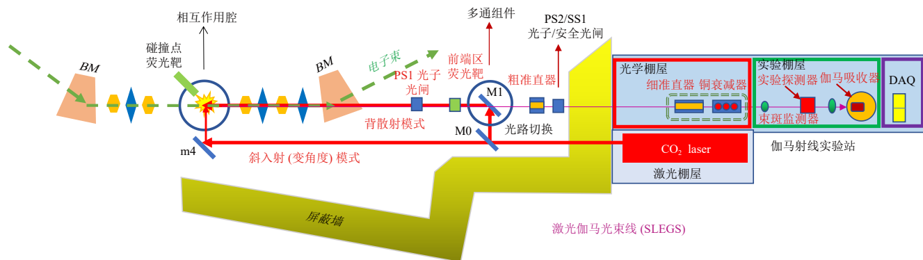
图 1 SLEGS 装置布局示意图
