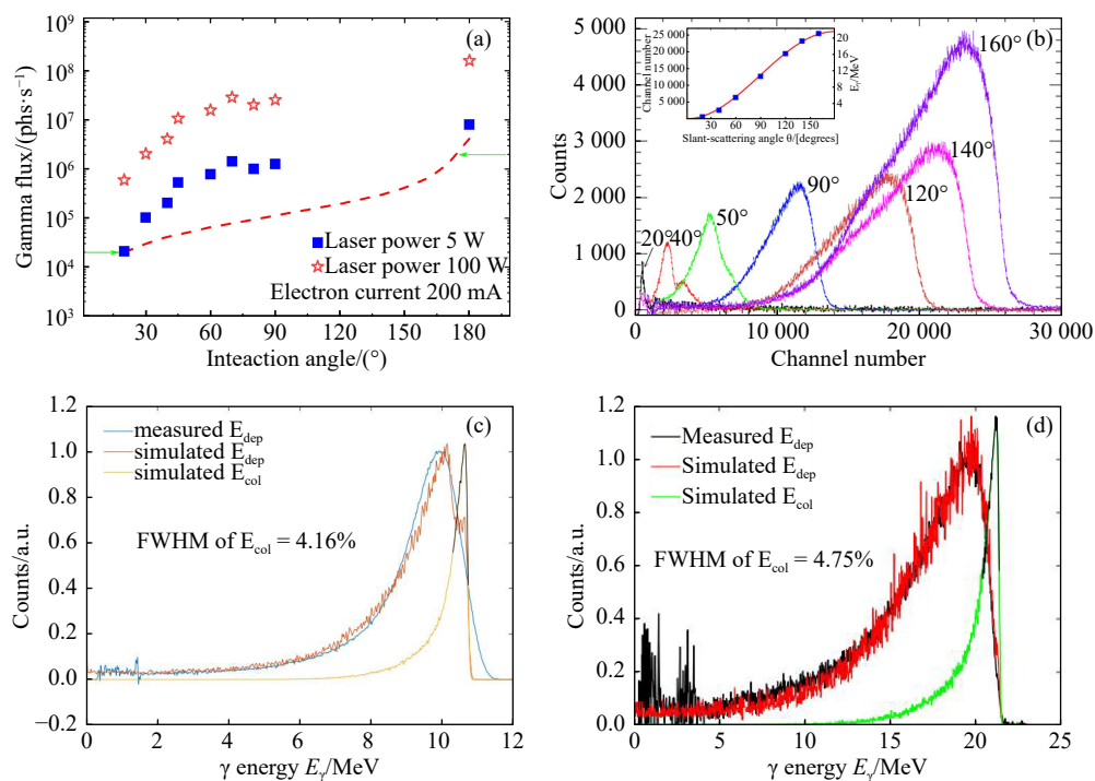
图5 SLEGS测试运行中测量的通量与能谱分析, 分别对应(a)伽马产额分布、(b)不同角度下伽马能谱、(c)90°伽马能谱解谱和(d)180°伽马能谱解谱(在线彩图)
