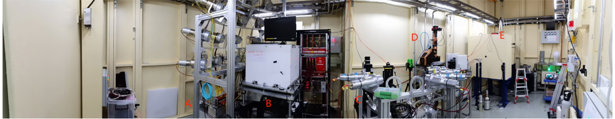
图4 SLEGS实验棚屋的TOF和FED谱仪现场照片(广角镜头拍摄,从左到右分别为A:飞行时间谱仪TOF支架和EJ301闪烁体探测器, B:平坦效率谱仪FED支架及电子学机柜, C:核共振荧光谱仪NRF的部分溴化镧探测器及支架, D:束斑监测器(MiniPIX和GSM)以及E:伽马束流垃圾桶)
