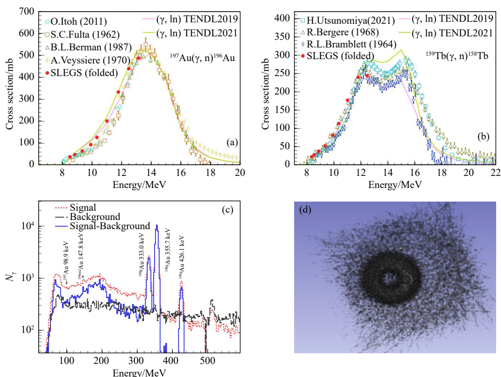
图 6 SLEGS 测试运行中的 (a)、(b) 光中子截面测量, (c) 伽马活化分析及 (d) 伽马成像谱分析 (对中空铅坠的成像)
