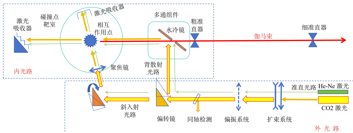
图 2 SLEGS 的光路系统示意图 (分为内光路和外光路两部分)
