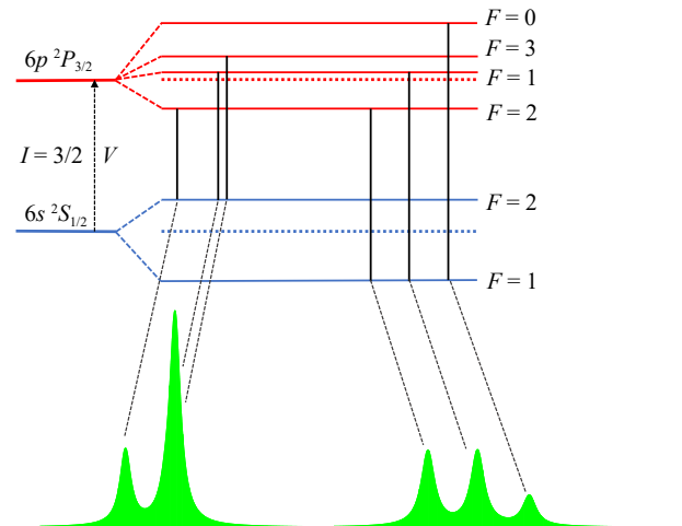
图 1 自旋为 I=3/2 的 ^{197}\text{Au} 原子 6s^2S_{1/2} 和 6p^2P_{3/2} 能级的超精细能级分裂，以及相应跃迁的超精细结构谱
