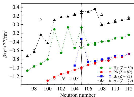
图 3 Pb 区域缺中子核素的均方电荷半径(在线彩图) 其中实心点表示基态, 空心点表示同核异能态 [51] 。
