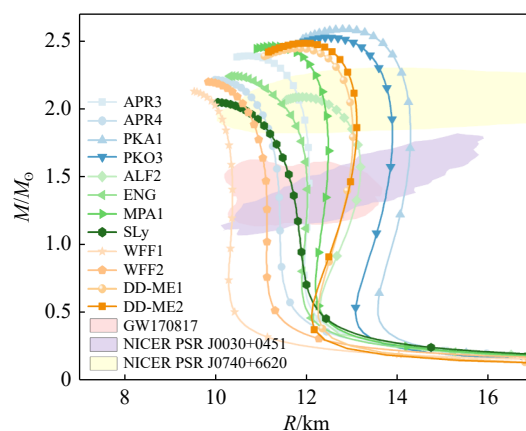
图 1 十二组物态 M - R 关系图(在线彩图)
