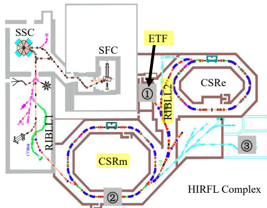
图 1 HIRFL 平面布局示意图(在线彩图)
