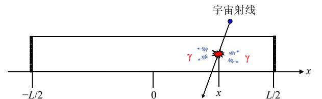
图 4 宇宙射线击中单元条示意图
