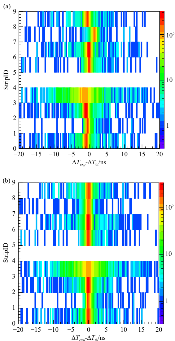
图 7 Veto 探测器 \Delta T_{\text{exp}} - \Delta T_{\text{th}} 在修正前 (a) 与修正后 (b) 的分布图
