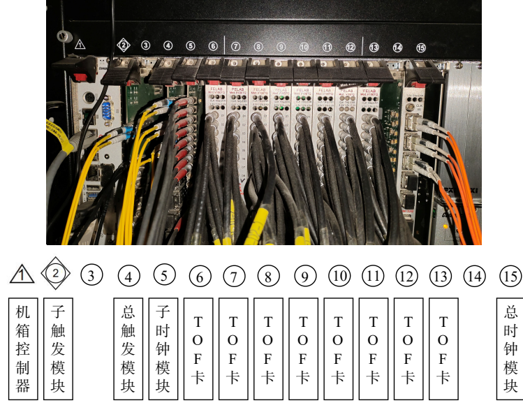
图 3 PXI 机箱及其插件
