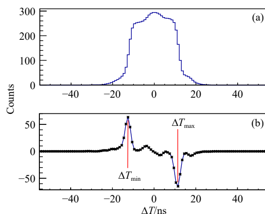
图 5 (a) 为 \Delta T 分布直方图, (b) 为 (a) 的计数变化率谱
