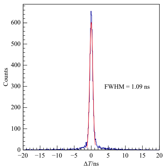
图 8 Veto 探测器时间分辨
