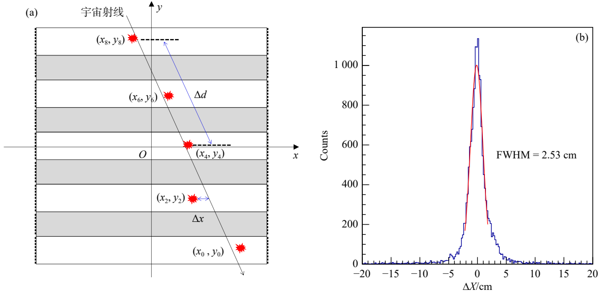
图 6 (a)为宇宙射线径迹拟合图, (b)为 Veto 探测器 x 方向位置分辨图
