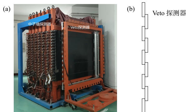
图 2 (a)为 ETF 中子墙探测器与 Veto 探测器实物图, (b)为 Veto 探测器侧视结构示意图
