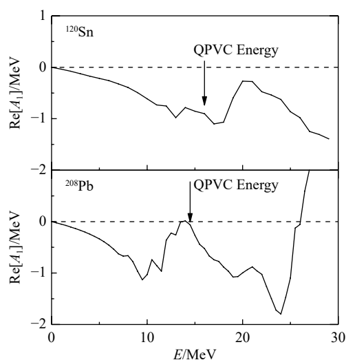
图 6 ^{120}\text{Sn} 和 ^{208}\text{Pb} 中 QPVC 方程自能 A_1(E) 的实部随能量的变化, 采用的相互作用为 SV-K226, 取自文献[46]
