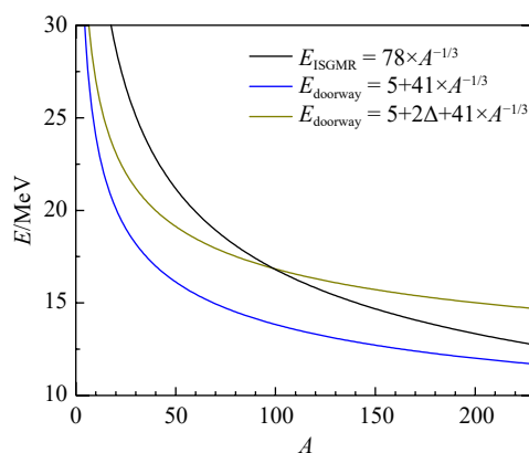
图 7 ISGMR 能量 E_{\text{ISGMR}} 的经验公式随质量数 A 的变化, 和中间态能量 E_{\text{doorway}} 近似公式在包含和不包含对关联效应时随质量数 A 的变化, 取自文献[46]
