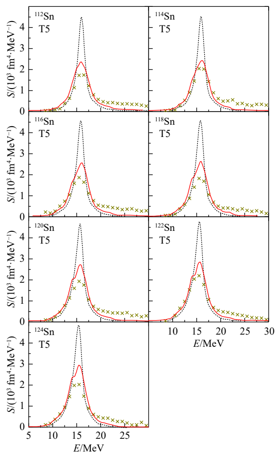
图 3 采用 Skyrme T5 相互作用参数, 基于 QRPA 和 QRPA+QPVC 理论计算的 Sn 同位素链 ISGMR 强度分布 (在线彩图)
