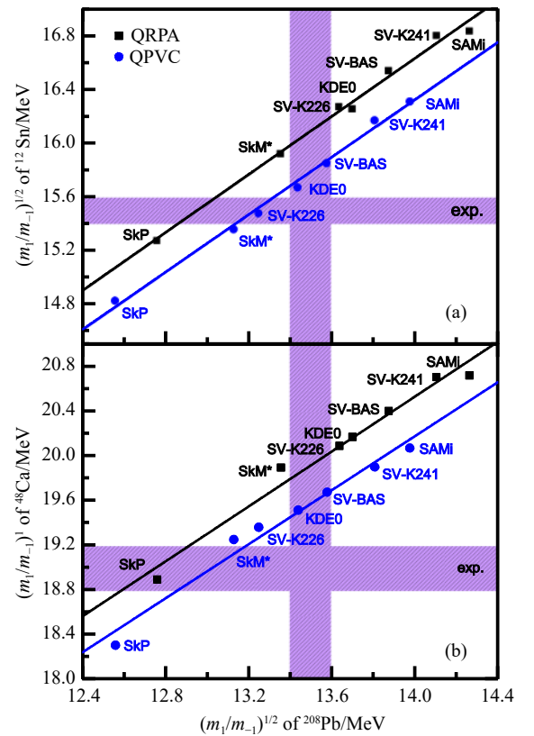
图 5 ^{120}\text{Sn} (a)、 ^{48}\text{Ca} (b) 中 ISGMR 能量和 ^{208}\text{Pb} ISGMR 能量的关系, 取自文献 [46] (在线彩图)
