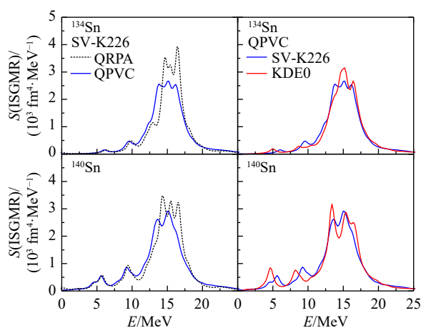
图 10 基于 QRPA 和 QRPA+QPVC 理论采用 SV-K226 相互作用计算的 ^{134, 140}\text{Sn} 中电单极激发强度分布 (左图) 和基于 QRPA+QPVC 理论采用 SV-K226 和 KDE0 相互作用计算的 ^{134, 140}\text{Sn} 中电单极激发强度分布 (右图)
