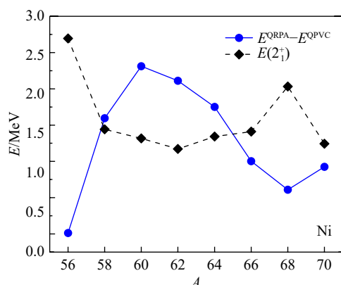
图 9 采用 NL3* 相互作用 QPVC 效应带来的 Ni 同位素链中 ISGMR 能量的移动 E^{\text{QRPA}} - E^{\text{QPVC}} 和实验上第一个 2_1^+ 激发能 E(2_1^+) 随着质量数的变化 (相关结果取自文献 [59])
