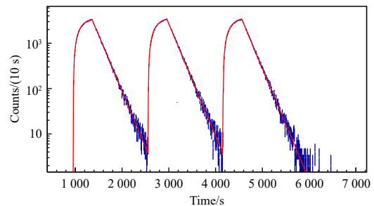
图7 利用LAMBDA-II原位 \beta^+ 测量得到的 ^{14}\text{N}(\text{p}, \gamma)^{15}\text{O} 反应 259 \text{ keV} 共振产物的衰变时间谱(在线彩图)
