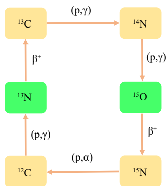
图1 CNO循环氢燃烧过程
