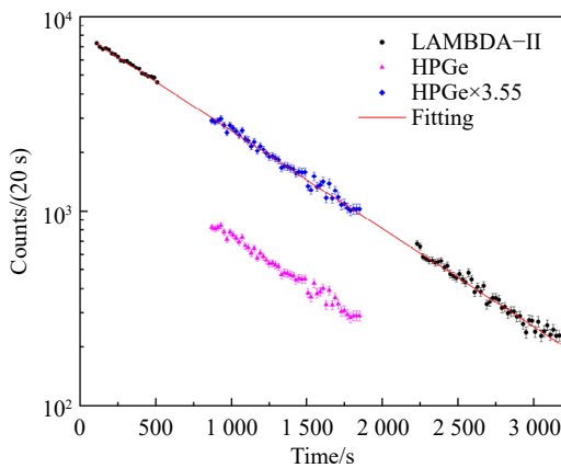
图6 停束后 ^{12}\text{C}(\text{p}, \gamma)^{13}\text{N} 反应产物 ^{13}\text{N} 的 \beta^+ 衰变曲线(在线彩图)
