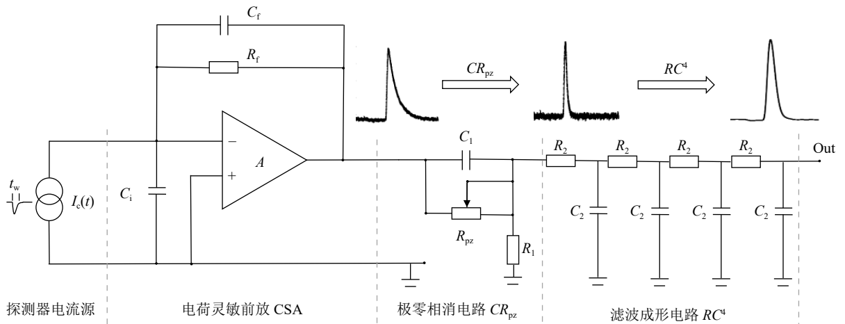
图 5 电荷灵敏前放- CR_{pz} - RC^4 电路与对应的 \alpha 放射源信号处理图
