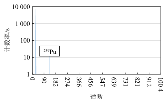
图 8 ^{239}\text{Pu} 空白样品 200 s 的测量能谱
