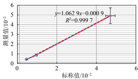
图 9 239 Pu 系列标准样品测量值与标称值的关系图
