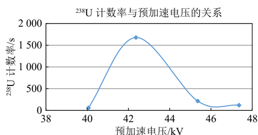
图 5 ^{238}\text{U} 计数率与预加速电压关系
