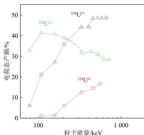
图3 不同能量的 ^{238}\text{U} 经氦气剥离后的电荷态分布 [18]
