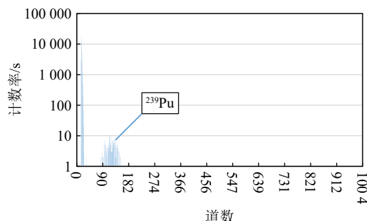
图 7 ^{239}\text{Pu} 标准样品 30 s 测量能谱
